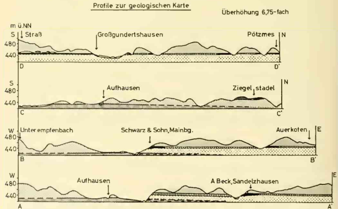
Abb. 4: Geologische Profile für den Südost-Quadranten des Gradabteilungsblattes 7336 Mainburg. Zur Lage der Profile vgl. Abb. 3. Geol. Aufnahme: J. GREGOR, 1969.
