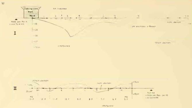
Abb. 7: Höhenlage und Verlauf der Fundschicht-Basis in der ehemaligen Kiesgrube KARBEN in Sandelzhausen: I) im Westteil der Grube (Bereich der Grabungsstellen West und Mitte), II) im Ostteil der Grube (Grabungsstelle Ost).
