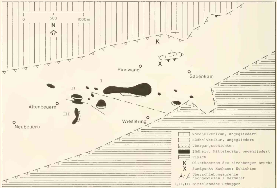
Abb. 2: Tektonische Übersichtsskizze des Helvetikums von Neubeuern am Inn mit besonderer Berücksichtigung des südhelvetischen Mitteleozäns
