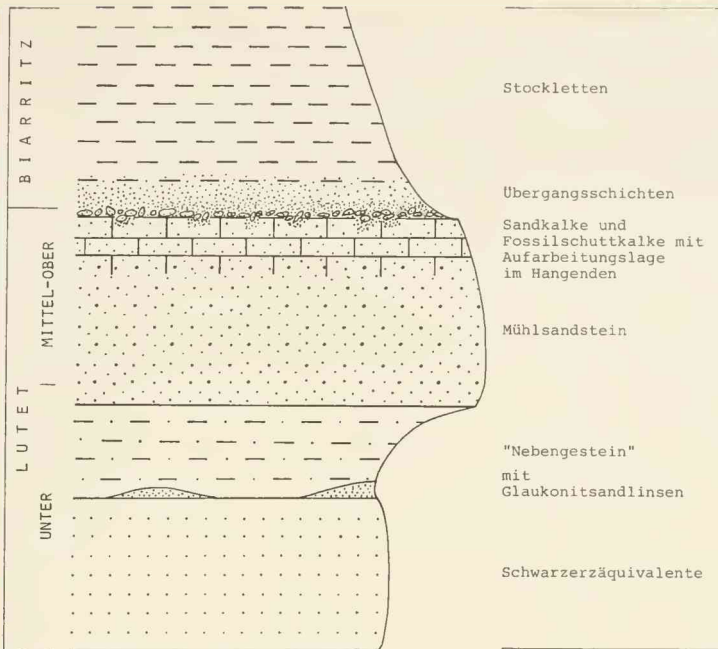
Abb. 1: Stratigraphisches Gliederungsschema des südhelvetischen Miozäns im Raum Neu- beuern-Hinterhör (Einheit II)
