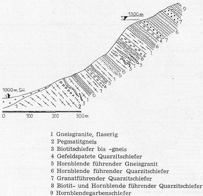
Profil 2: Der Verband zwischen Gneisgranit und Hornblendequarzitschieferserie im Raum Sachersee Alm (SE) — Säulecksockel (NW)
