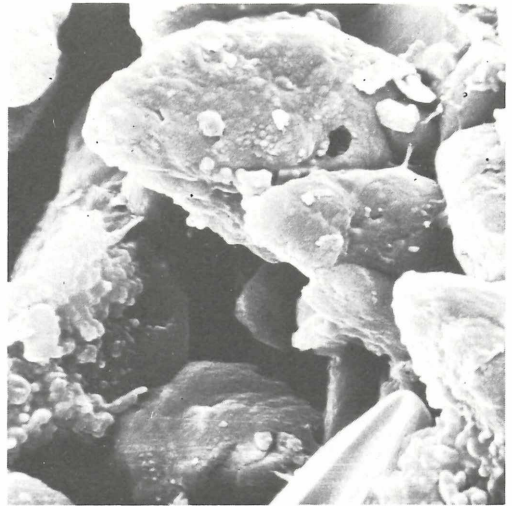
Abb. 10: Rim-Zement aus Hoch-Mg-Kalzit mit vertikalen und horizontalen Hohlräumen ehemals organischer Diatomeen-Halbefäden. Im oberen Bilddrittel zwei Diatomeen-Frusteln. REM-Foto 2-4665; Probe Rarotonga 6; Vergrößerung 1400x.
