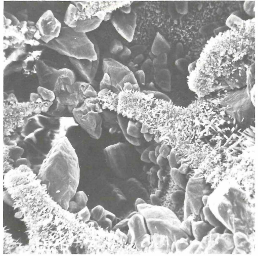
Abb. 6: Hoch-Mg-Kalzit-Skalenoedern als Zement in Halimeda-Hohlräumen. REM-Foto 2-4479; Probe Rarotonga 4; Vergrößerung 770x.
