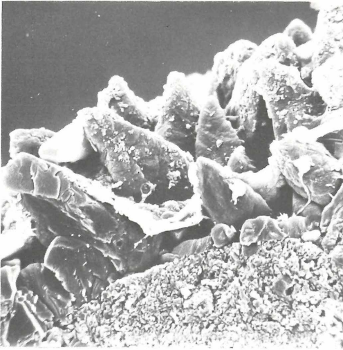
Abb. 5: Rim-Zement aus Hoch-Mg-Kalzit-Skalenoedern um ein Halimeda-Fragment. REM-Foto 2-4477; Probe Rarotonga 4; Vergrößerung 1500x.
