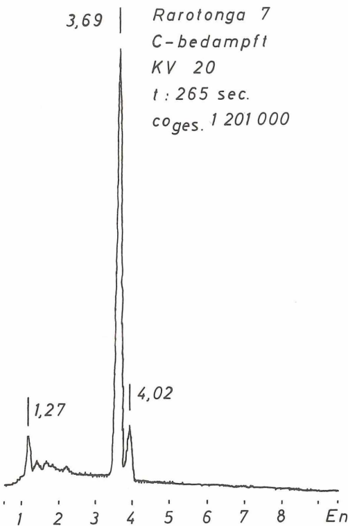
Abb. 4: Diagramm der Mikroanalyse skalenoedrischer Beachrock-Zemente von Rarotonga, das mit Hilfe eines röntgenenergie-dispersiven Systems (ORTEC) erstellt wurde. Zählzeit: 265 sec; Gesamtcounts: 1 201 000; Beschleunigungsspannung: 20 KV. Die Peaks bei folgenden Emissionsenergien (in keV) entsprechen: 1,27 : Mg (K \alpha ), counts max. : 1965 3,69 : Ca (K \alpha 1 +2), counts max. : 16 338 4,02 : Ca (K \beta 1), counts max. : 2413 Aus dem Peakverhältnis Ca : Mg läßt sich in grober Annäherung ein Molanteil von ca. 11-12% MgCO 3 ermitteln; ein Wert, der Hoch-Mg-Kalzit belegt.
