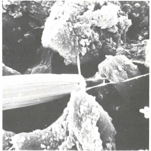
Abb. 8: Frustel einer benthonisch lebenden Kieselalge mit ihren organischen Haltefäden, die von Hoch-Mg-Kalzit umwachsen werden. REM-Foto 2-4640; Probe Rarotonga 6; Vergrößerung 4000x.
