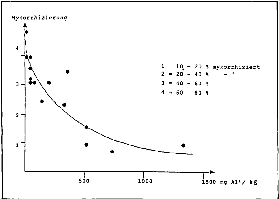
Abbildung 2: Zusammenhang zwischen austauschbarem Al (1 M KCl) und Mykorrhizierung von Buchenfeinwurzeln im A-Horizont von Braunlehmern (n = 40) am Gaisberg.
