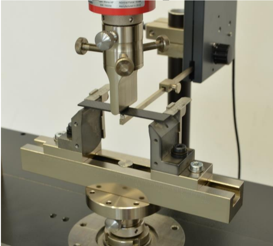
3-Punkt Biegeversuch
